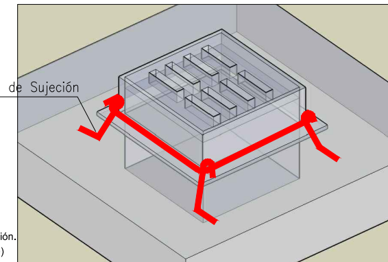
Detalle anclaje de marco y tapa
