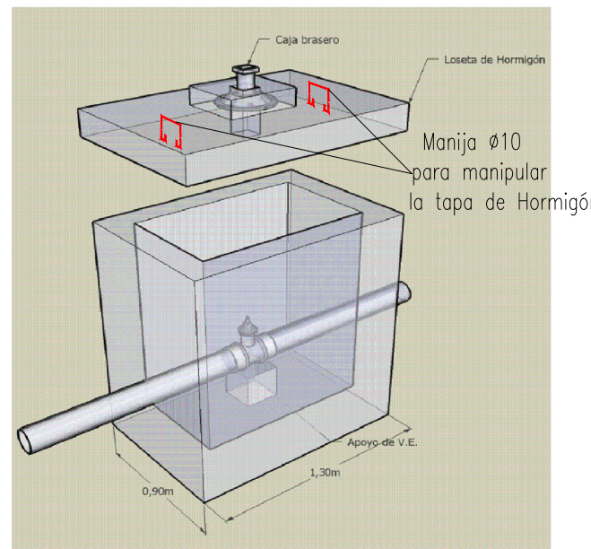
Detalle anclaje de caja brasero
