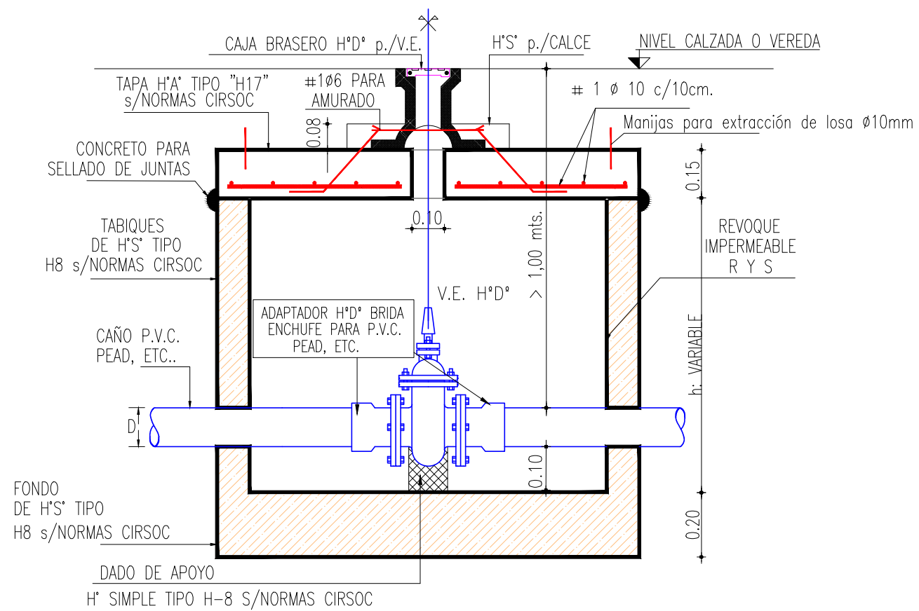
CORTE A-A
