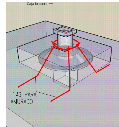
Detalle de armadura en loseta superior
