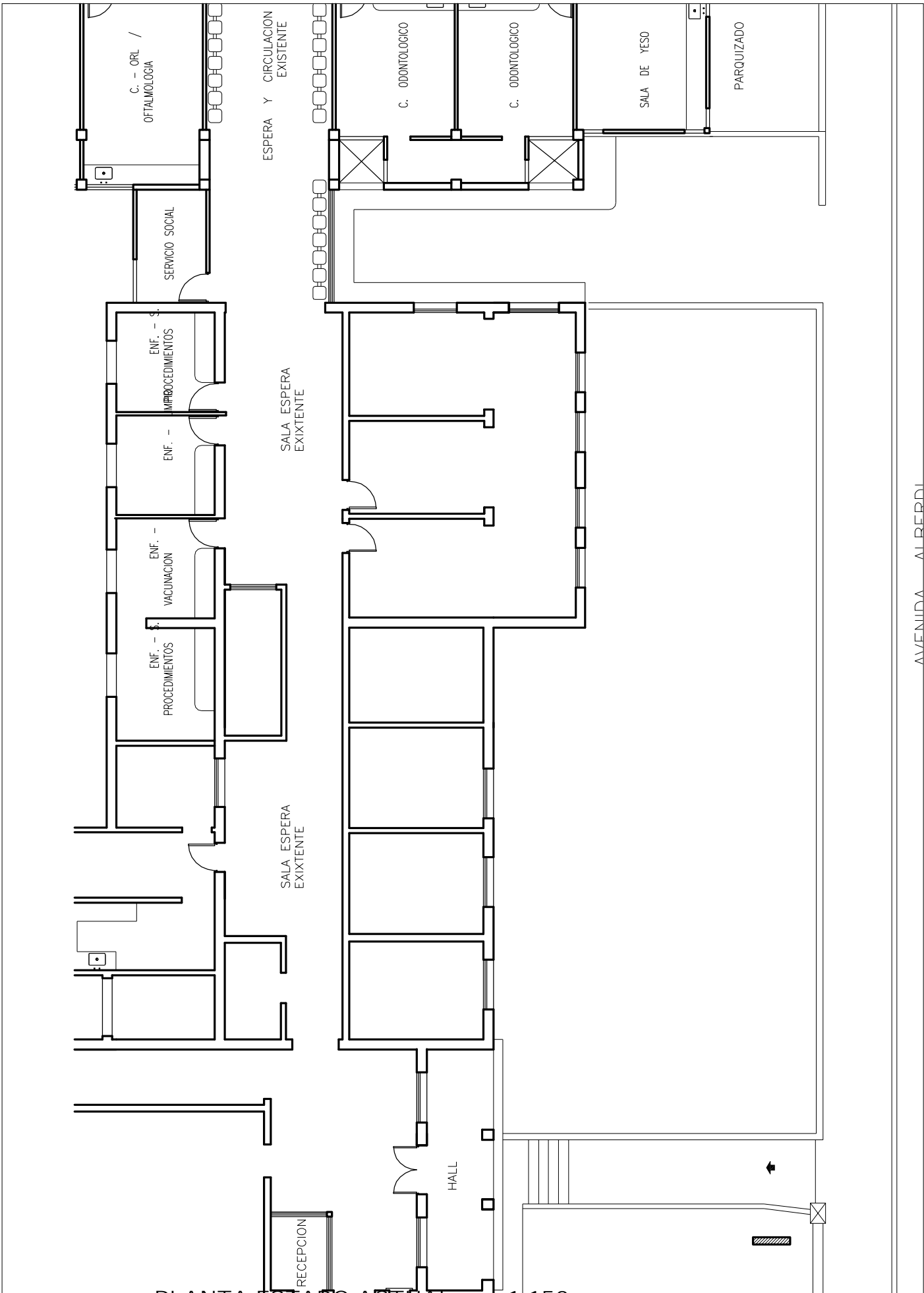
PLANTA ESTADO ACTUAL esc 1:150
